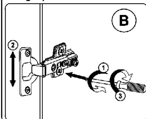
Регулировка петель
