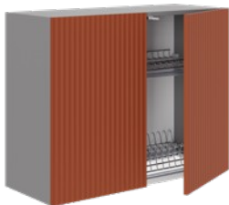
ШСВ-800_Н6 (800 x 626 x 314 мм)
