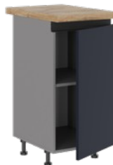
C-300 (300 x 820 x 478 мм) C-350 (350 x 820 x 478 мм) C-400 (400 x 820 x 478 мм) C-450 (450 x 820 x 478 мм) C-500 (500 x 820 x 478 мм) C-550 (550 x 820 x 478 мм) C-600 (600 x 820 x 478 мм)
