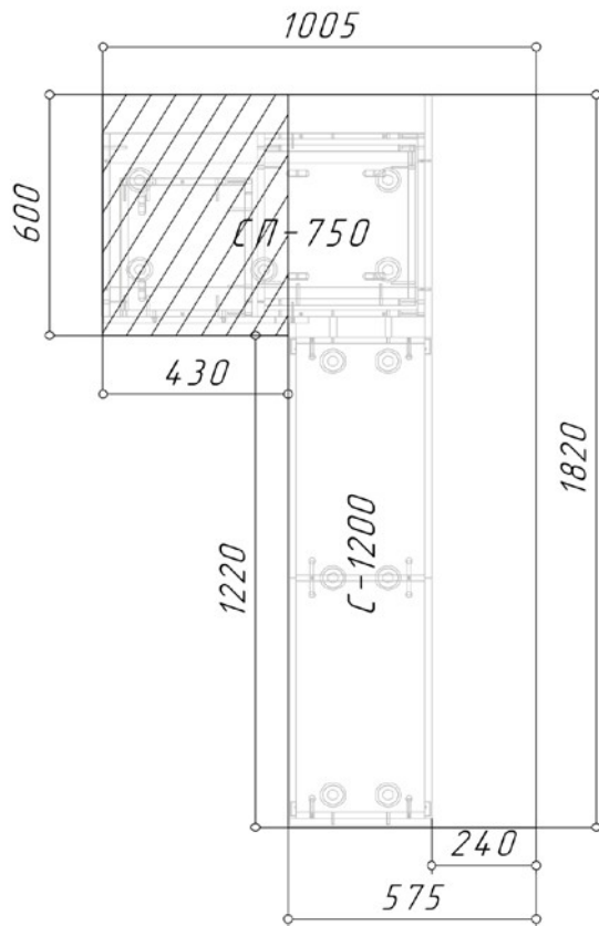
Расчетные размеры столешницы для острова (модули С-1200 + СП-750)
