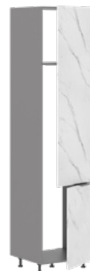
ПХВ-400_H10 (400 x 2425 x 570 мм)
