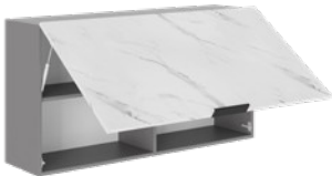
Г-1200_Н6 (1200 x 626 x 315 мм)
